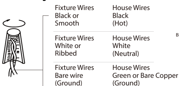
FIG. 3 Wiring
