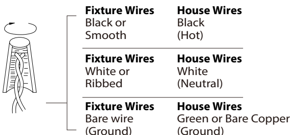
Fig. 2 Wiring
